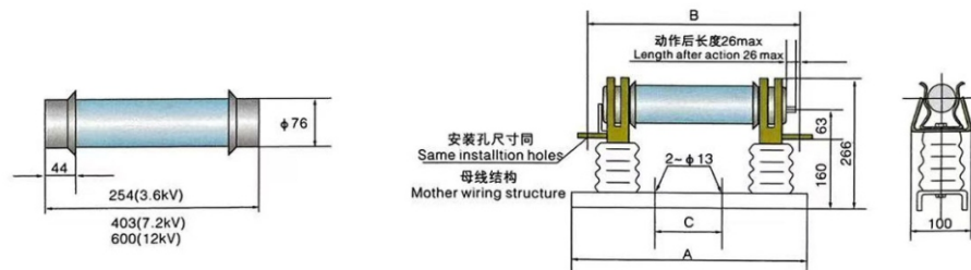
图2 插入式熔断器外形及安装尺寸 Chart 2 Inserting fuse Lnstallation Dimensions
