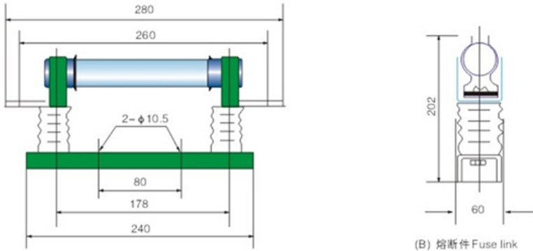
XRNP底座尺寸图 (XRNP base size diagram)
