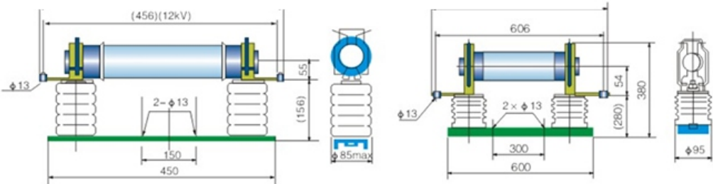
XRNT底座尺寸图 (XRNT base size diagram)
