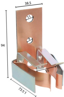
RN卡子 (RN Card)
