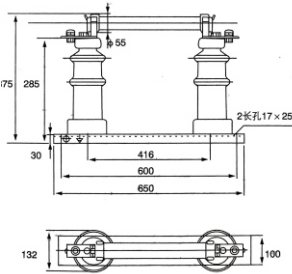
RN2-15、20/2-0.5型外形尺寸 RN2-15、20/2-0.5 External dimensions of the type
