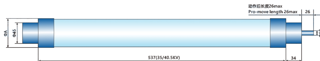
熔断器Char1/a link XRNT□-35/40.5KV
