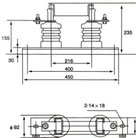
RN2-3、6、10/0.5型外形尺寸 RN2-3、6、10/0.5 External dimensions of the type
