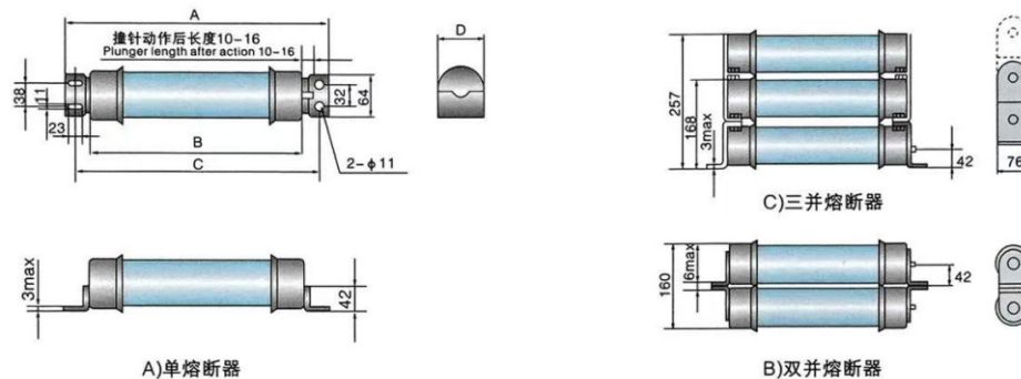
图1 母线式熔断器外形及安装尺寸 Chart 1 Generatrix fuse Lnstallation Dimensions
