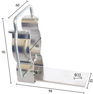
RN卡子 (RN Card)
