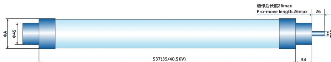
熔断器Char1/a link XRNT□-35/40.5KV
